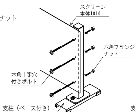
スクリーン1010 H=1000取付
