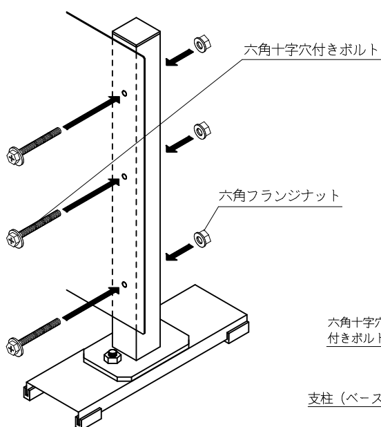
ボルト・ナット組付詳細
