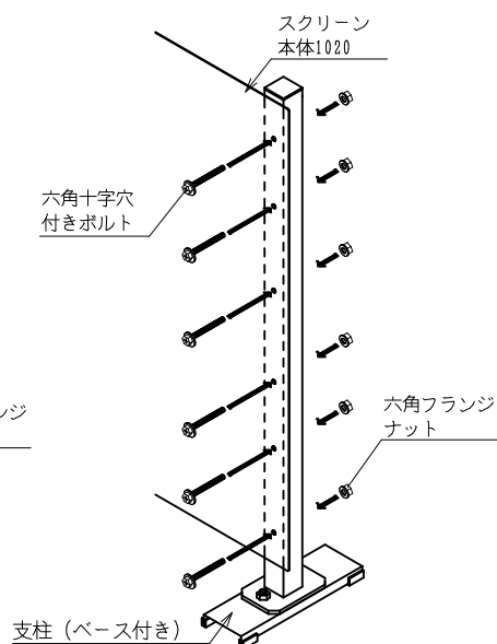
スクリーン1020 H=2000取付
