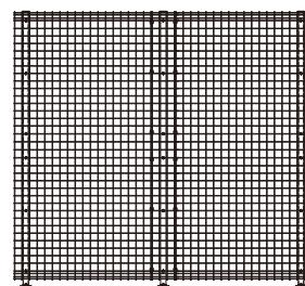
支柱H: 2000 (TCPT-0006)
